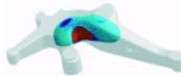
Bild 3: Darstellung der Erstarrungszeit zur Visualisierung der Wärmezentren.
